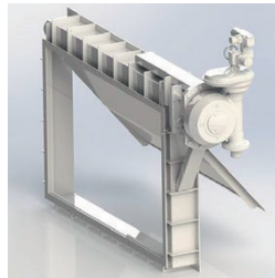
Kääntöpellit
